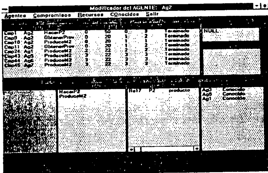
fig. 5.5 Estado mental final de un agente
